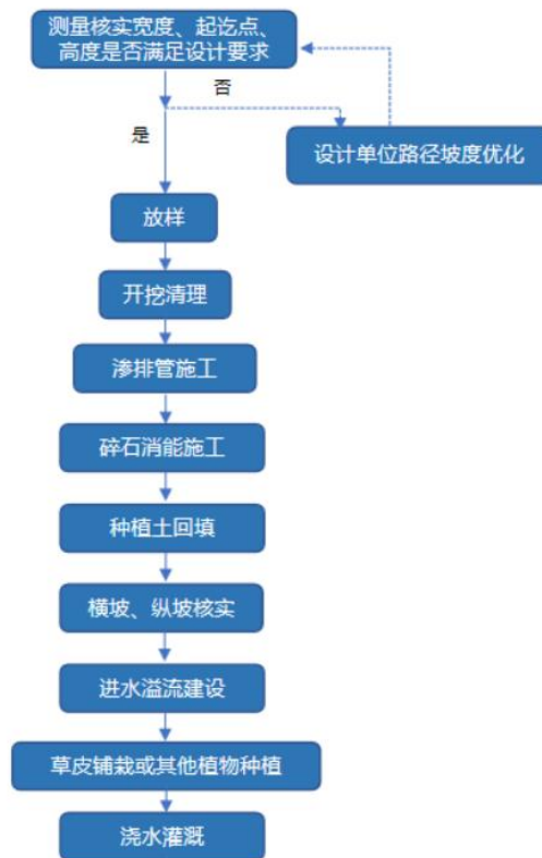
图 4.4-2 植被缓冲带施工工序
