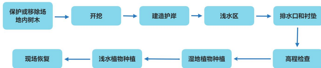
图 4.3-7 人工湿地施工步骤
