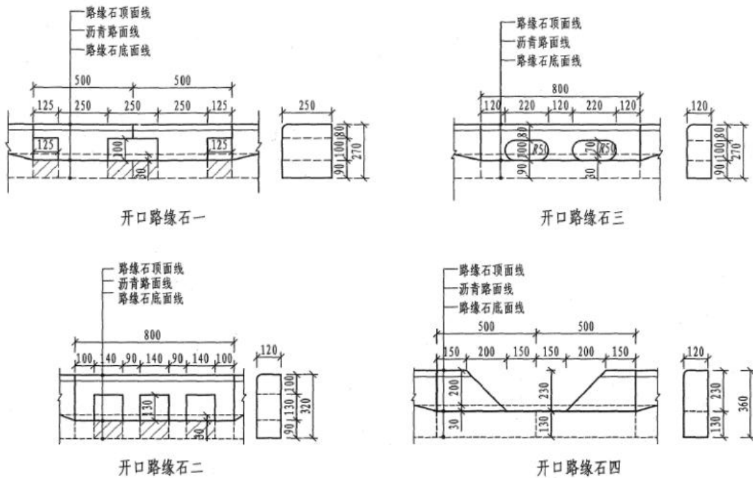
图 4.6-2 开口路缘石剖面图
