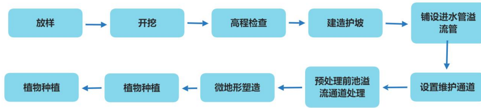
图 4.3-4 雨水塘施工步骤
