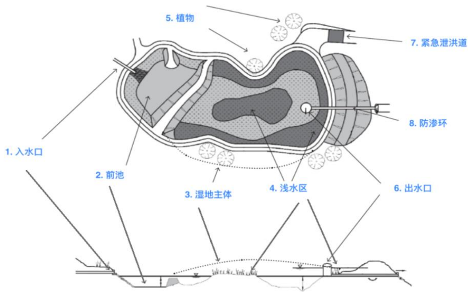
图 4.3-6 人工湿地组成部分
