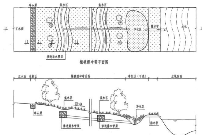
图 4.4-1 植被缓冲带平面/剖面图
