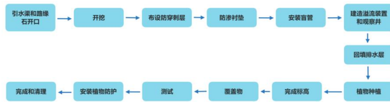
图 4.2-11 生态树池施工步骤
