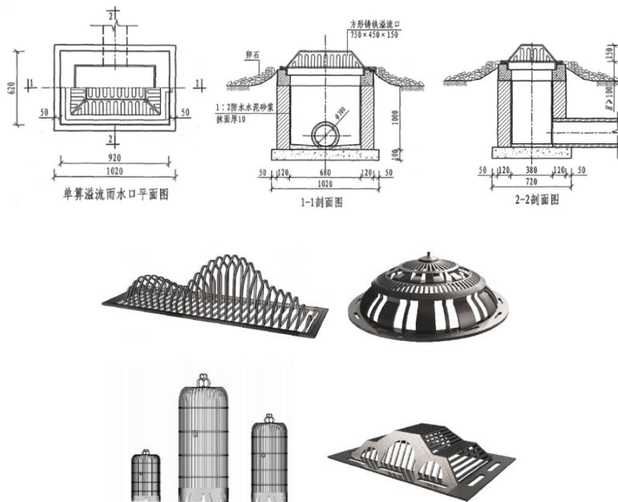
图 4.6-1 溢流井示意图
