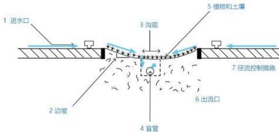
图 4.5-1 植草沟组成部分
