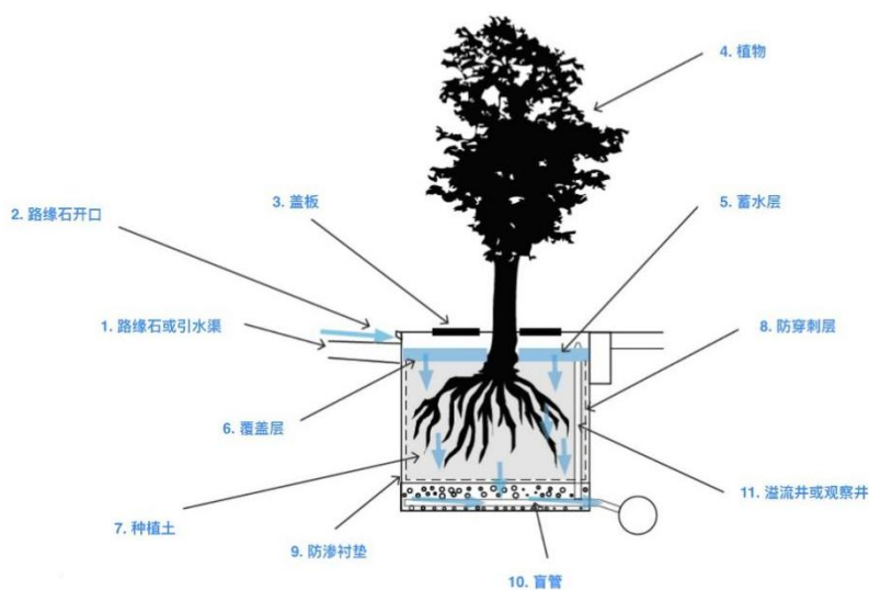
图 4.2-10 生态树池组成部分
