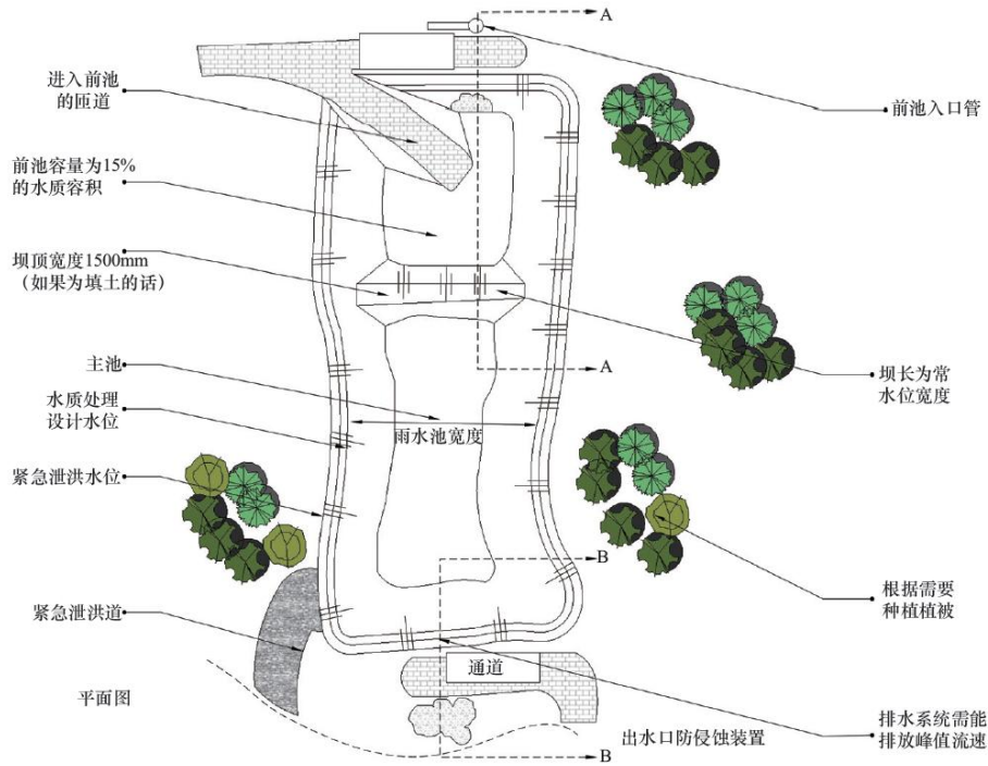
图 4.3-3 雨水塘平面图
