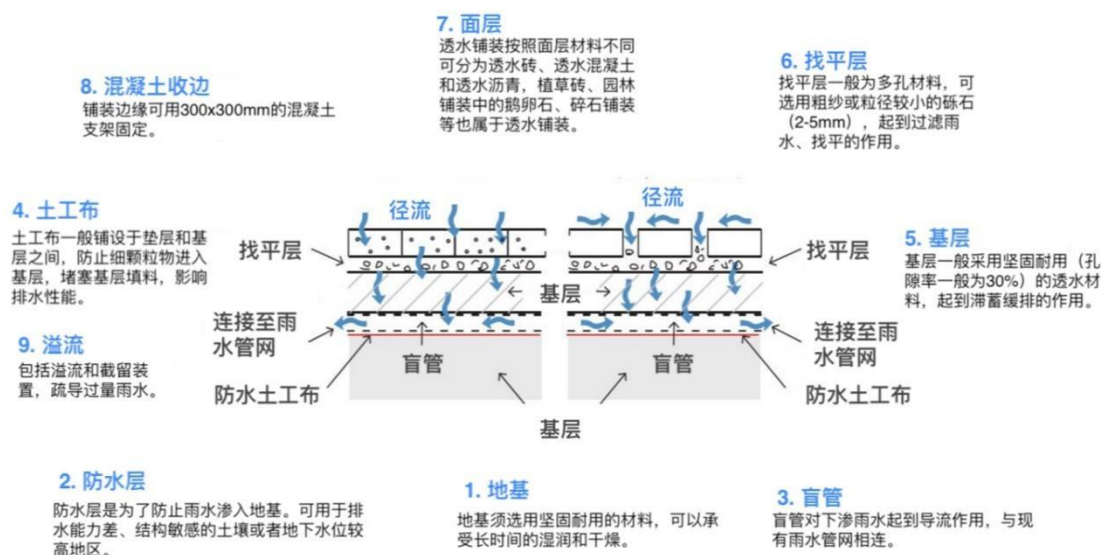
图 4.1-1 透水铺装的组成部分
