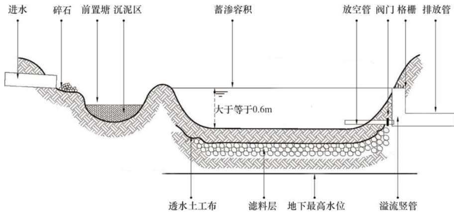
图 4.3-2 雨水塘剖面图
