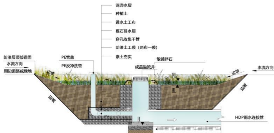
图 4.3-1 下凹式绿地组成部分
